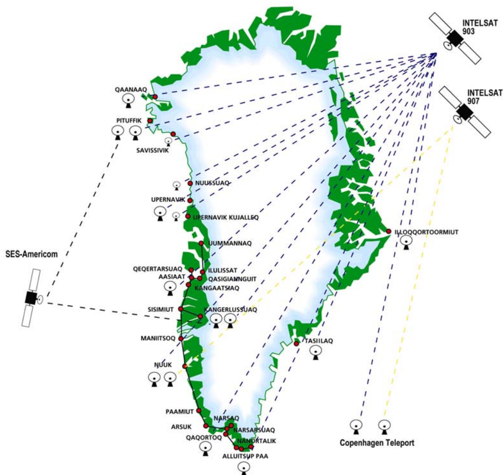
Ilusiligaq 3.1-1: TELE-p Kalaallit Nunaata iluani kiisalu Kalaallit Nunaannut tassanngaanniillu attaveqaateqarnikkut aqquersuutai pingaernerit
